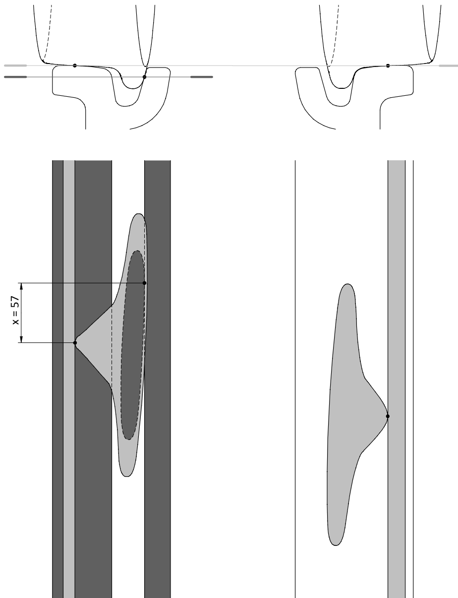
Obr. 4 Postavení dvojkolí v koleji při způsobu vedení dvojkolí přerubou vnitřní kolejnice (kolejnice typu NT1 R10 , rozchod koleje 1435 mm, úhel náběhu dvojkolí 2,72°, rozkolí 1379 mm, jízdní obrys DPMB-004)
