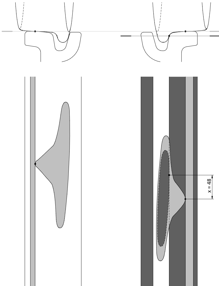
Obr. 3 Postaven  dvojkol  v koleji p i zp sobu veden  dvojkol  po jzdenou hranou vn j  i kolejnice (kolejnice typu NT1 R10 , rozchod koleje 1435 mm,  hel n b hu dvojkol  2,72 , rozkol  1380 mm, j zdn  obrys DPMB-004)
