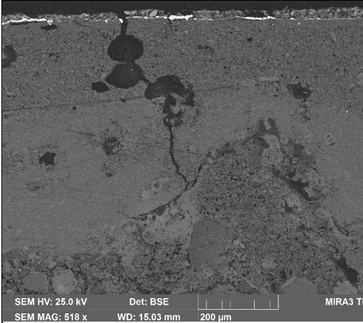
Obr. 59 Elektronová mikroskopie, BSE.
