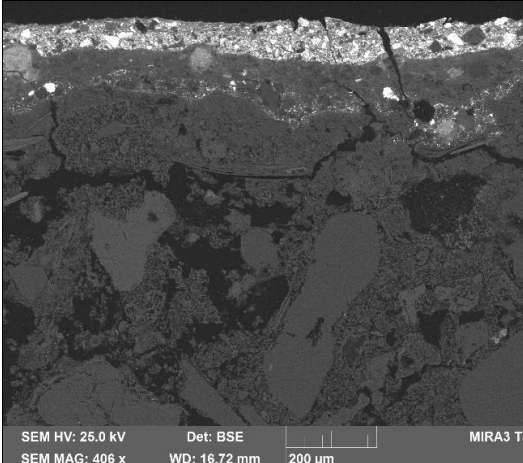
Obr. 26 Elektronová mikroskopie, BSE.
