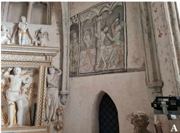
Záznam RTG dokumentace vnitřní konstrukce rámu výjevu oltáře sv. Šebestiána v kostele Nanebevzetí Panny Marie a svatého Václava ve Znojmě.
