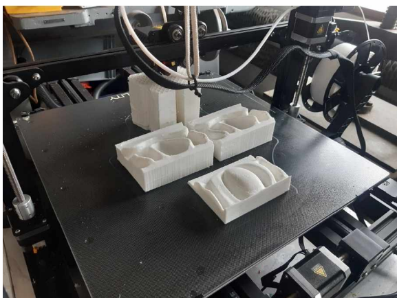
E) Tisk forem z PLA materiálu na tiskárně Creality CR-6 Max.
