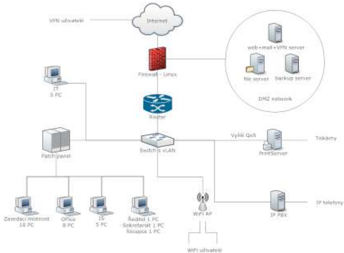
Obr. 1 - Topologie firemní sítě 1
