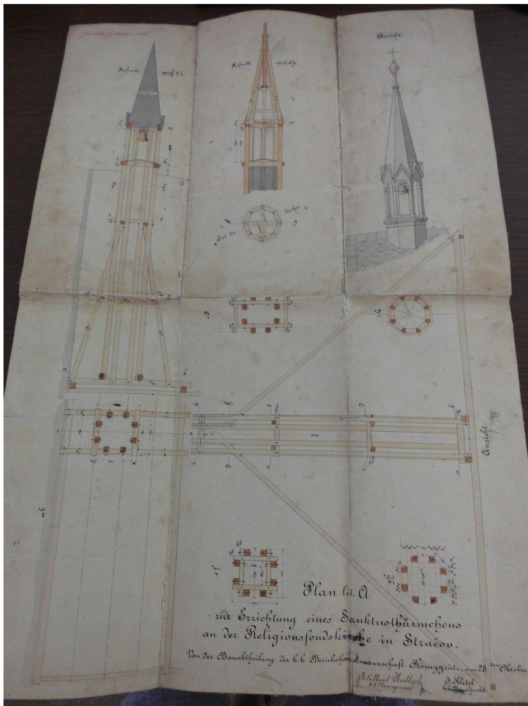
Plán na přestavbu kostelní věže ve Stračově
