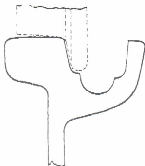
Obr. 1 Profil opotřeбенé pojezdové hrany žlábkové kolejnice
