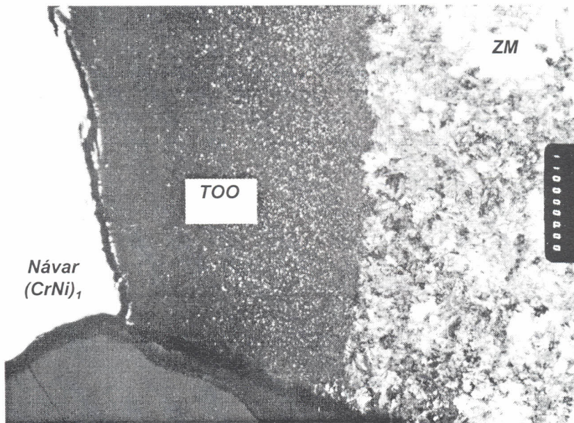
Obr. 8 Trhlina na hranici návar - kolejnice (zv. 63x)
