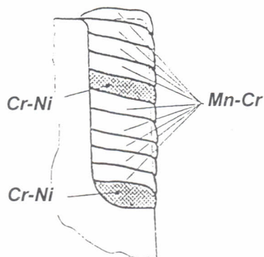
Obr. 2 Skladba navařených vrstev (MnCr tvrdonávar a CrNi mezivrstva)
