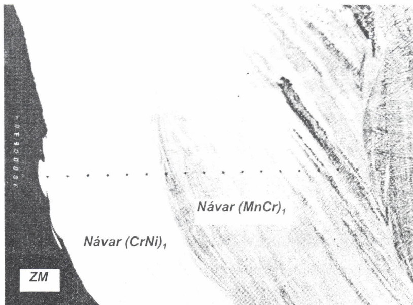
Obr. 11 Řada vpichů po měření mikrotvrdosti (zv. 63x)
