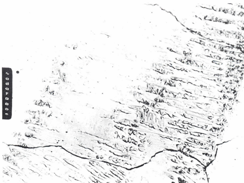
Obr. 14 Vlasové (tepelné) trhliny mezi sousedními zrny (zv. 400x)
