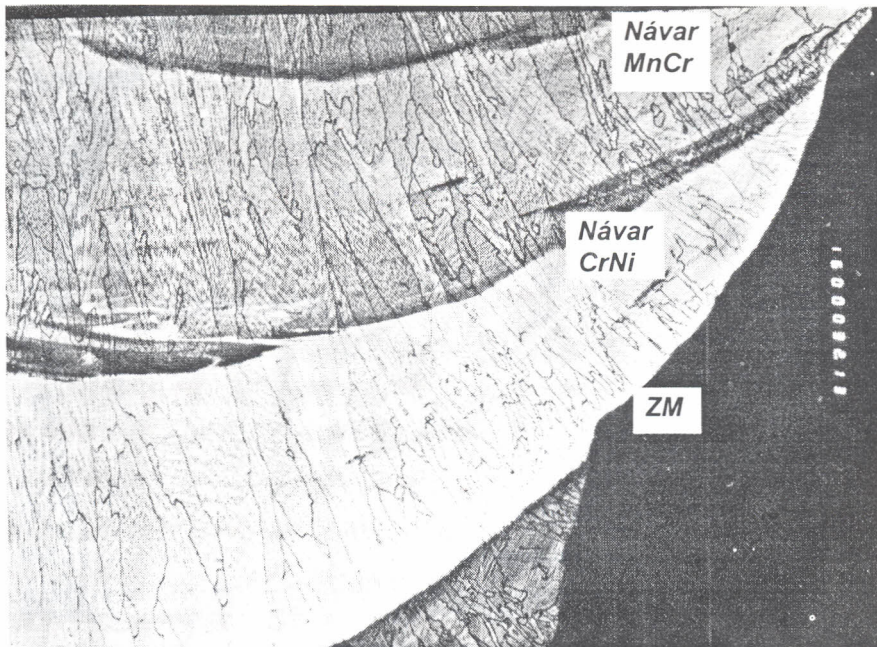
Obr. 12 Prorůstání dendritů jednotlivými návary (zv. 32x)
