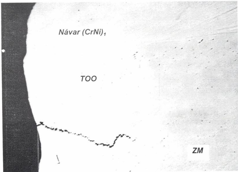
Obr. 6 Trhlina, vycházející z podnávarové oblasti (zv. 16x)
