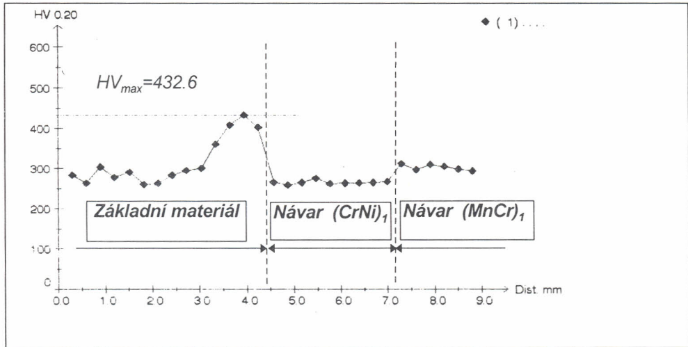
Obr. 7 Průběh mikrotvrdosti návarem a kolejnicí (viz umístění vpichů na obr. 9)
