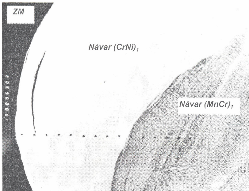
Obr. 9 Řada vpichů po měření mikrotvrlosti (zv. 63x)
