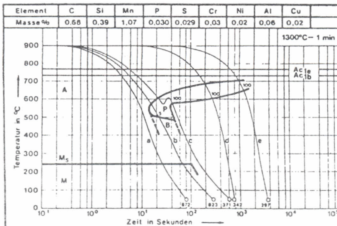
Obr. 3 Diagram rozpadu austenitu oceli UIC 900A
