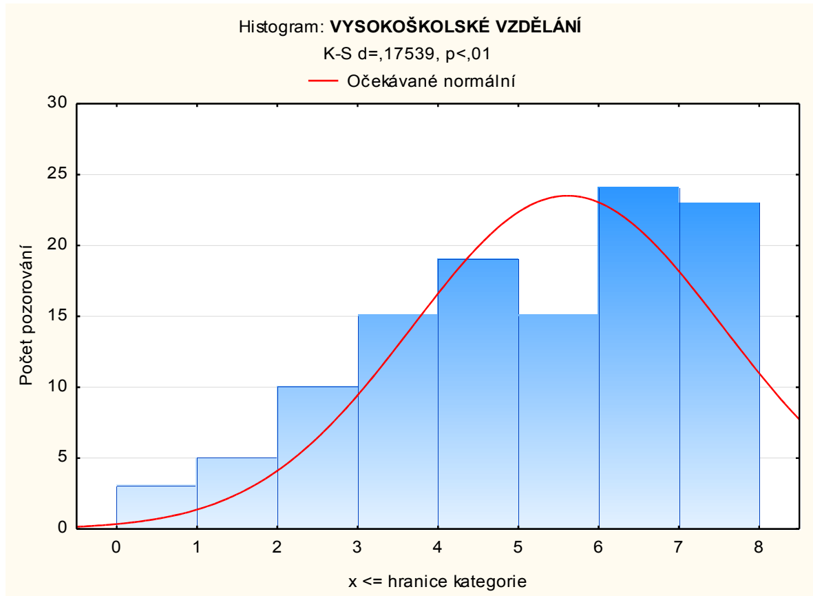
Graf 2 Histogram: vysokoškolské vzdělání
