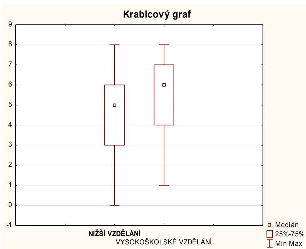
Graf 3 Krabicový graf: nižší vzdělání versus vysokoškolské vzdělání
