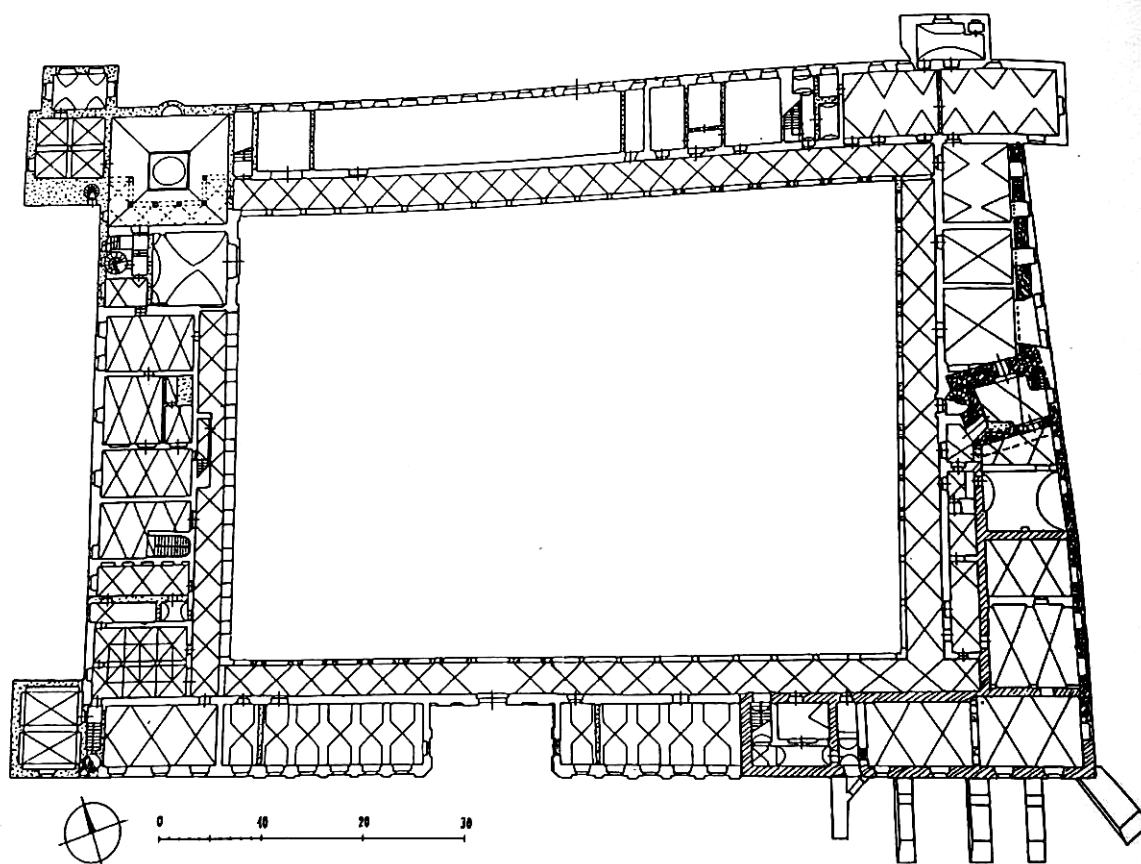
Obr.3/I Vývojové schéma zámku zrnitě je položeno starší gotické zdivo, šrafovaně pozdně gotické, tečkovaně barokní, ostatní (bíle) je renesanční (dle Plaček s.256 Podle B.Samek)
