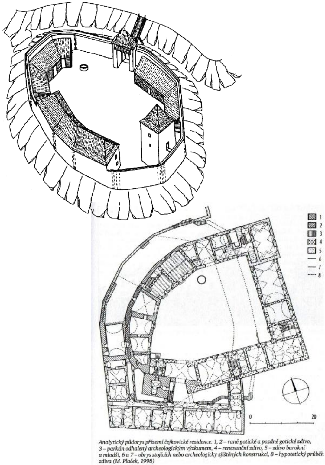
Půdorys přízemí komendy v Čejkovicích
