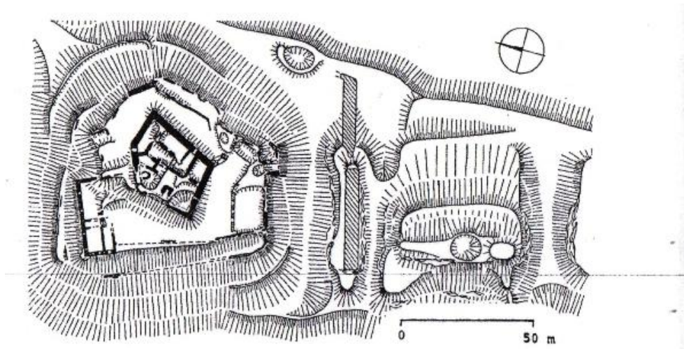
Terénní plán hradu Templštejn.
