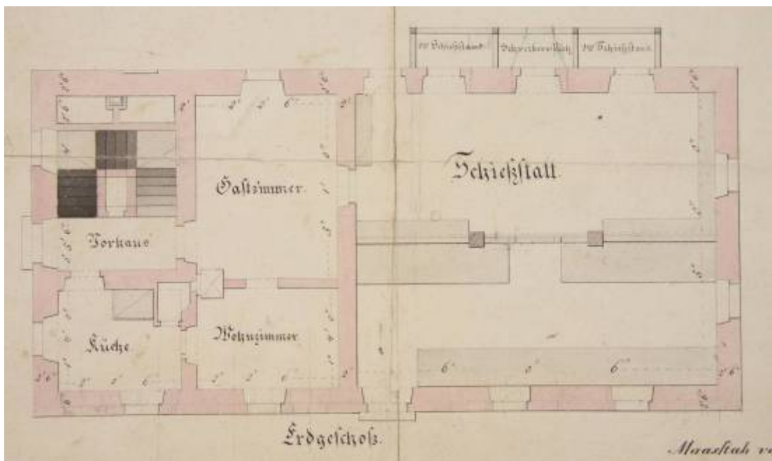
Obr. 14 Details plánu střelnice z roku 1837–přízemí a 1. patro
