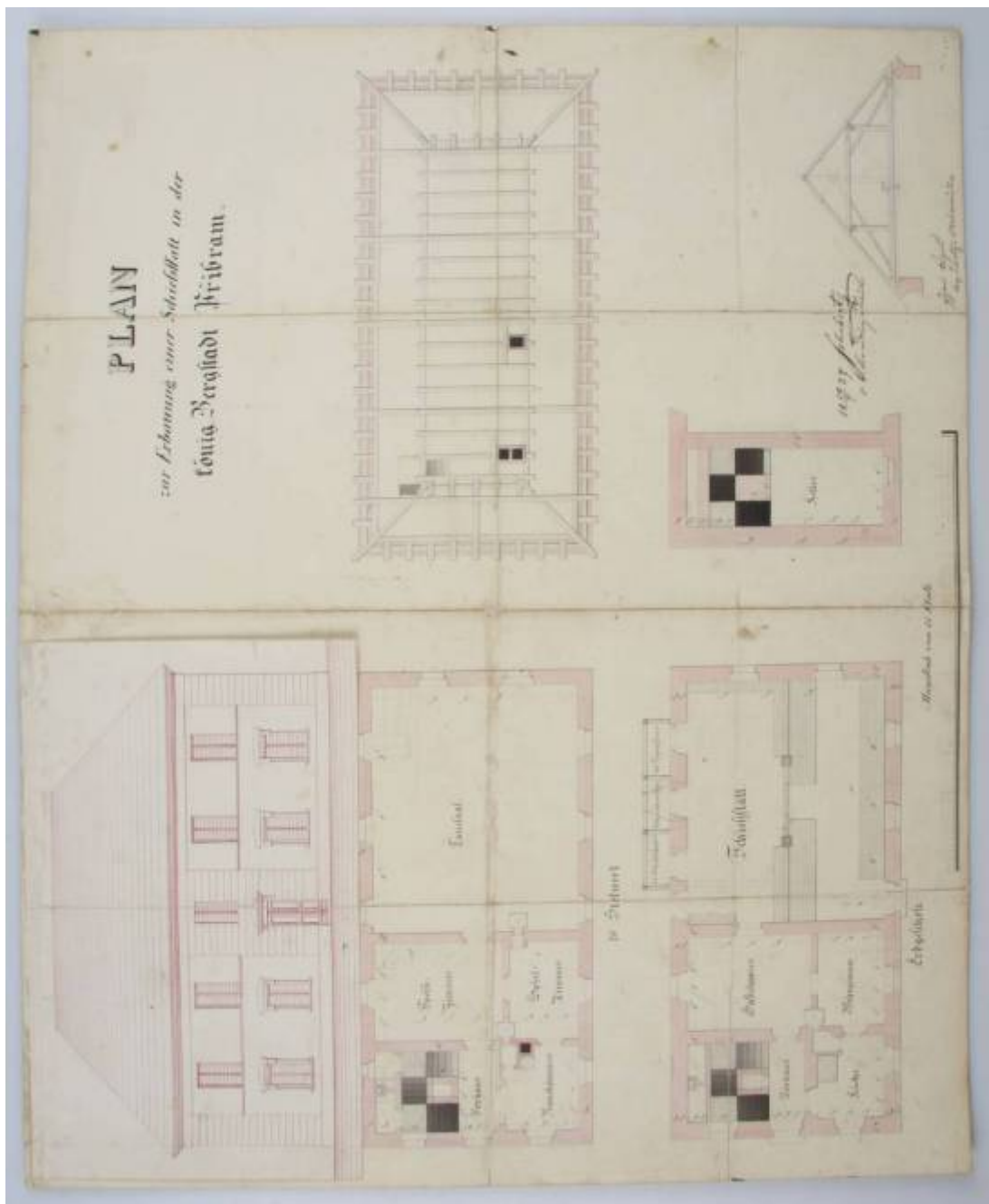
Obr. 13 Plán na výstavbu střelnice z roku 1837
