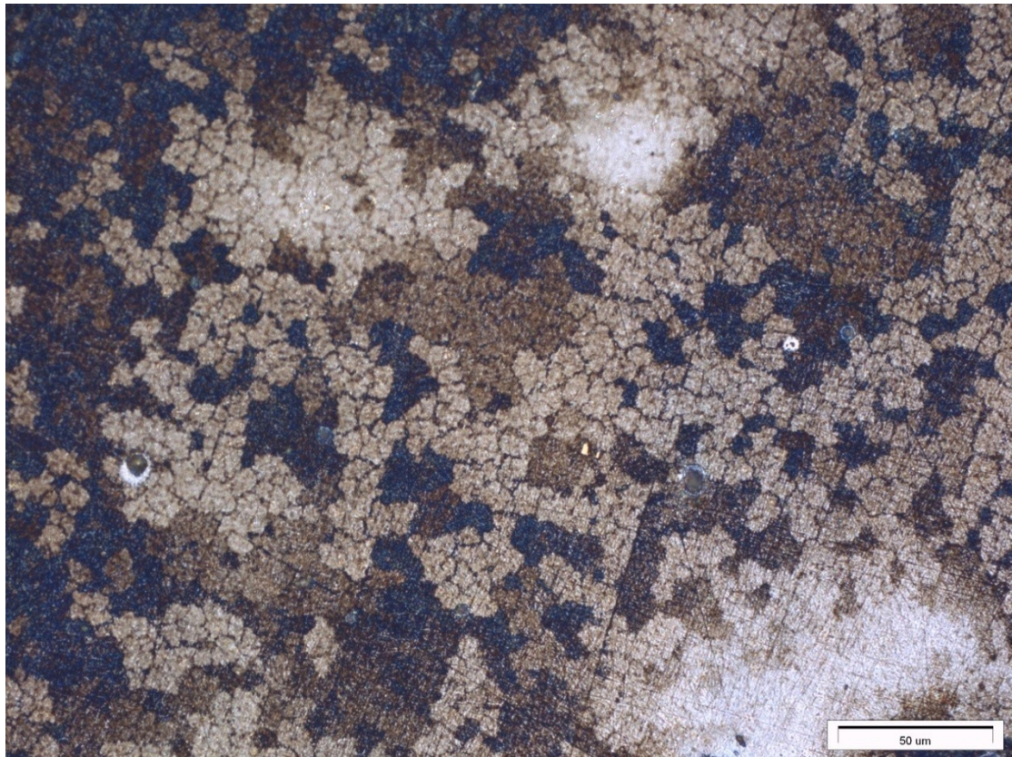
Obrázek: Perlit KLEMM (zvětšeno 400x)
