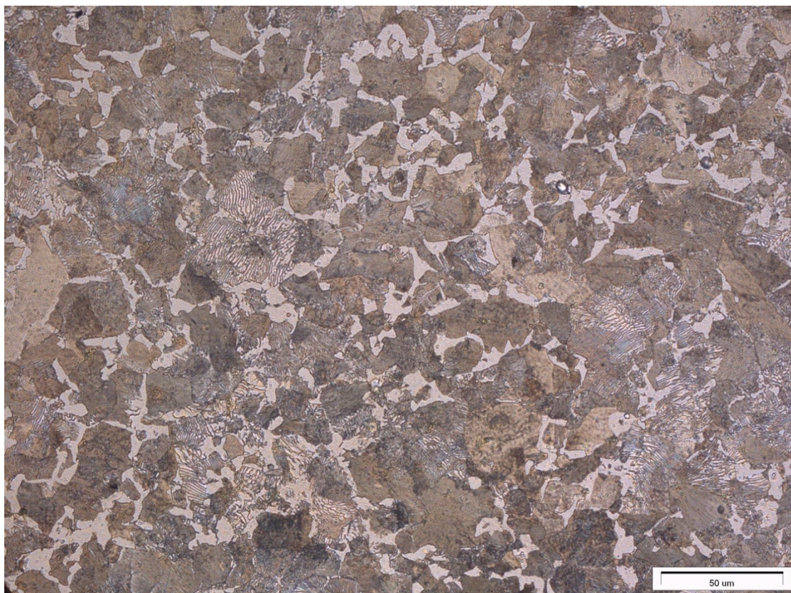
Obrázek: Perlit BERAHA I (zvětšeno 400x)
