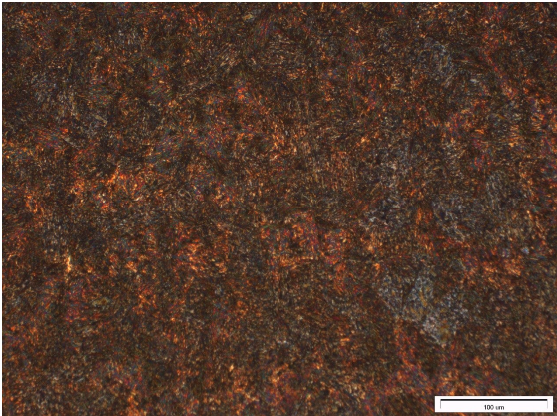
Obrázek: Tepelně zpracovaná ocel BERAHA-MARTENZIT (zvětšeno 250x)
