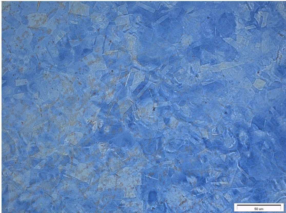
Obrázek: Austenitická ocel LICHTENEGGER A BLOECH I (zvětšeno 400x)
