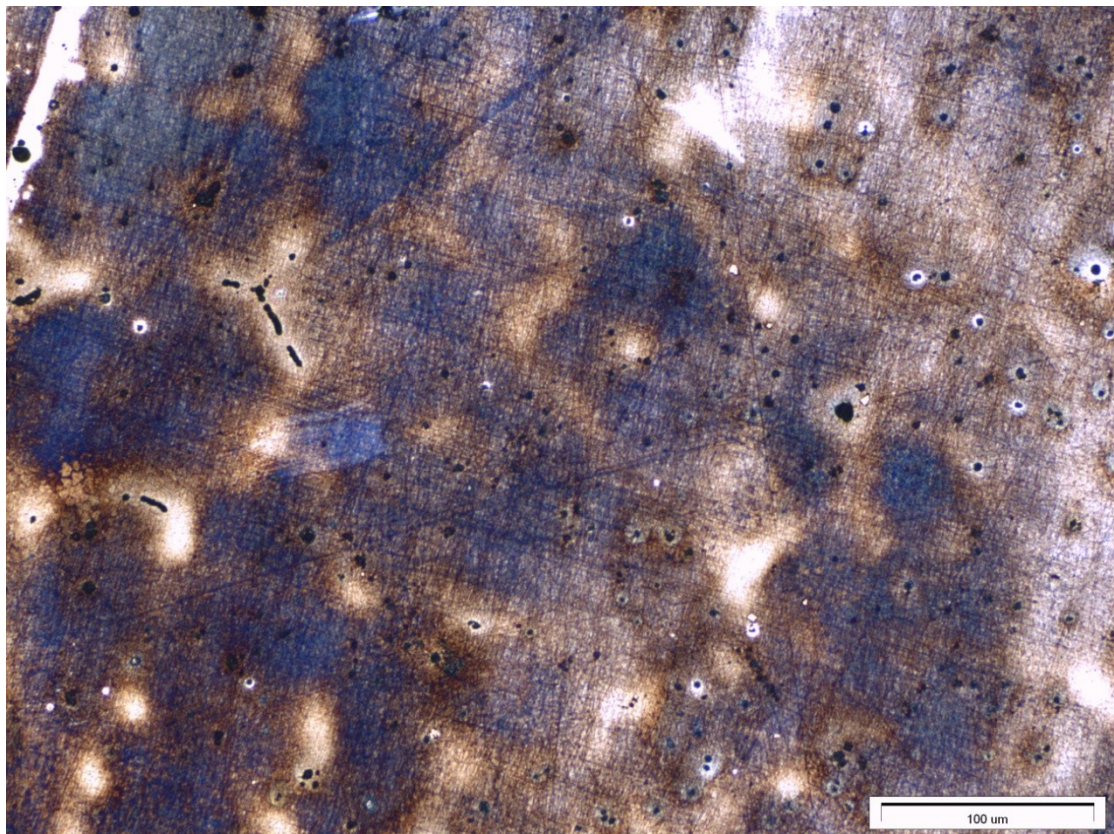
Obrázek: Perlit KLEMM (zvětšeno 250x)
