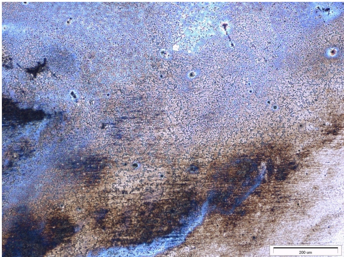
Obrázek: Perlit 2 KLEMM (zvětšeno 125x)
