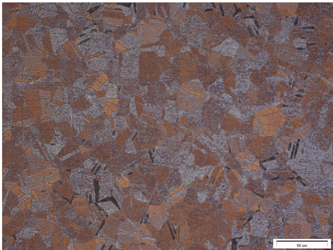
Obrázek: Austenitická ocel 2 BLOECH A WEDL I (zvětšeno 400x)
