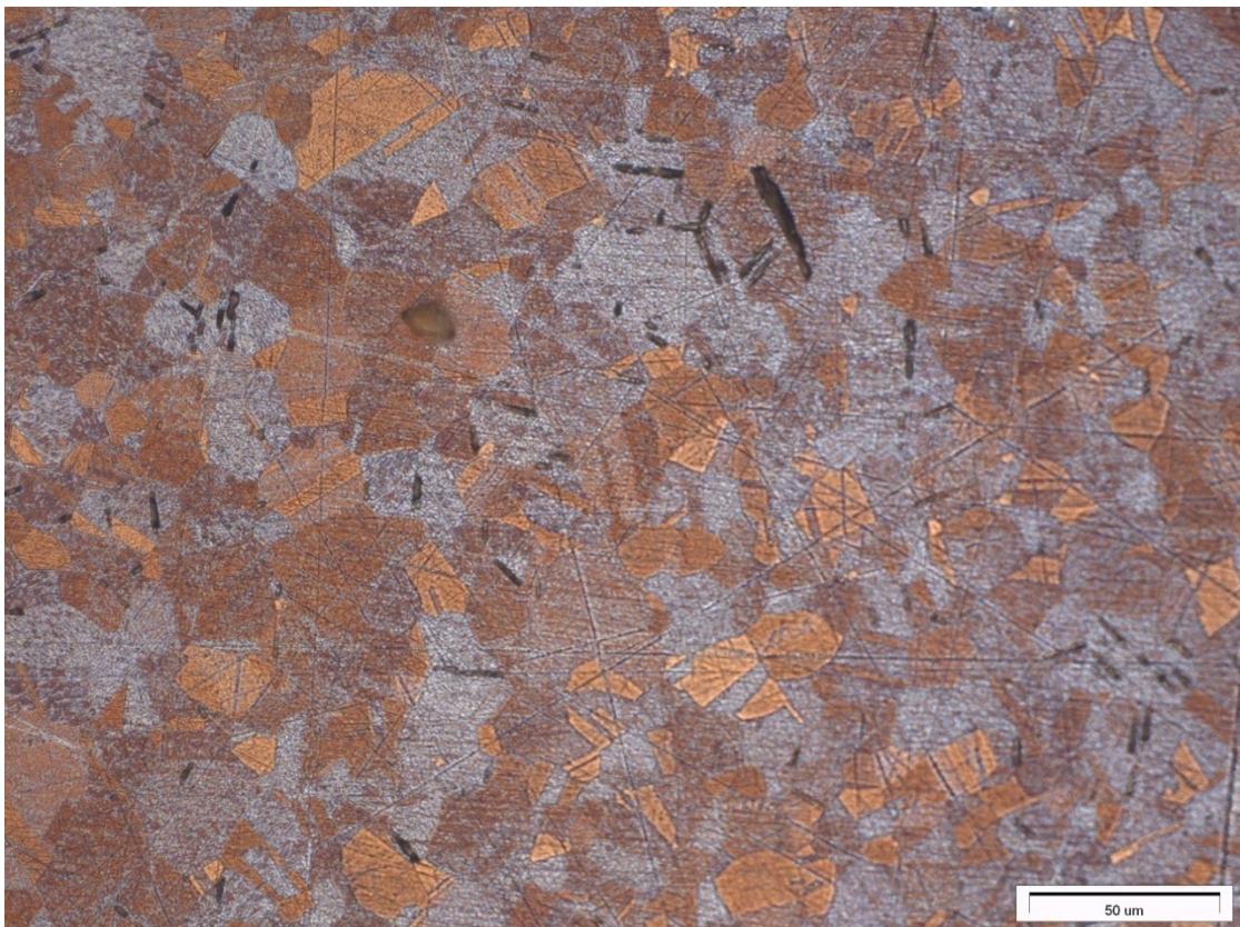
Obrázek: Austenitická ocel BLOECH A WEDL I (zvětšeno 400x)
