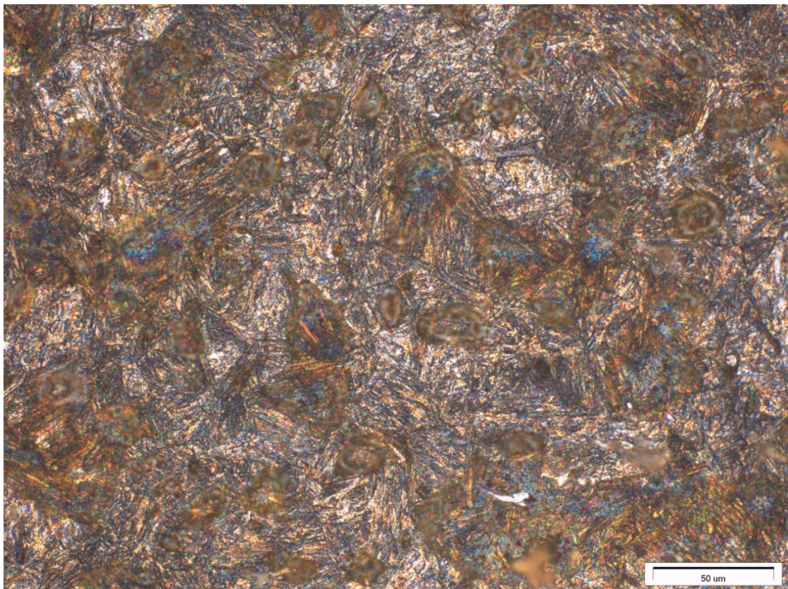
Obrázek: Tepelně zpracovaná ocel BERAHA II (zvětšeno 400x)
