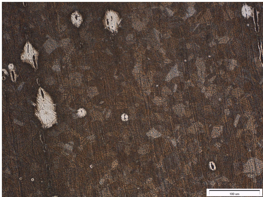
Obrázek: Austenitická ocel 2 BERAHA II (zvětšeno 250x)
