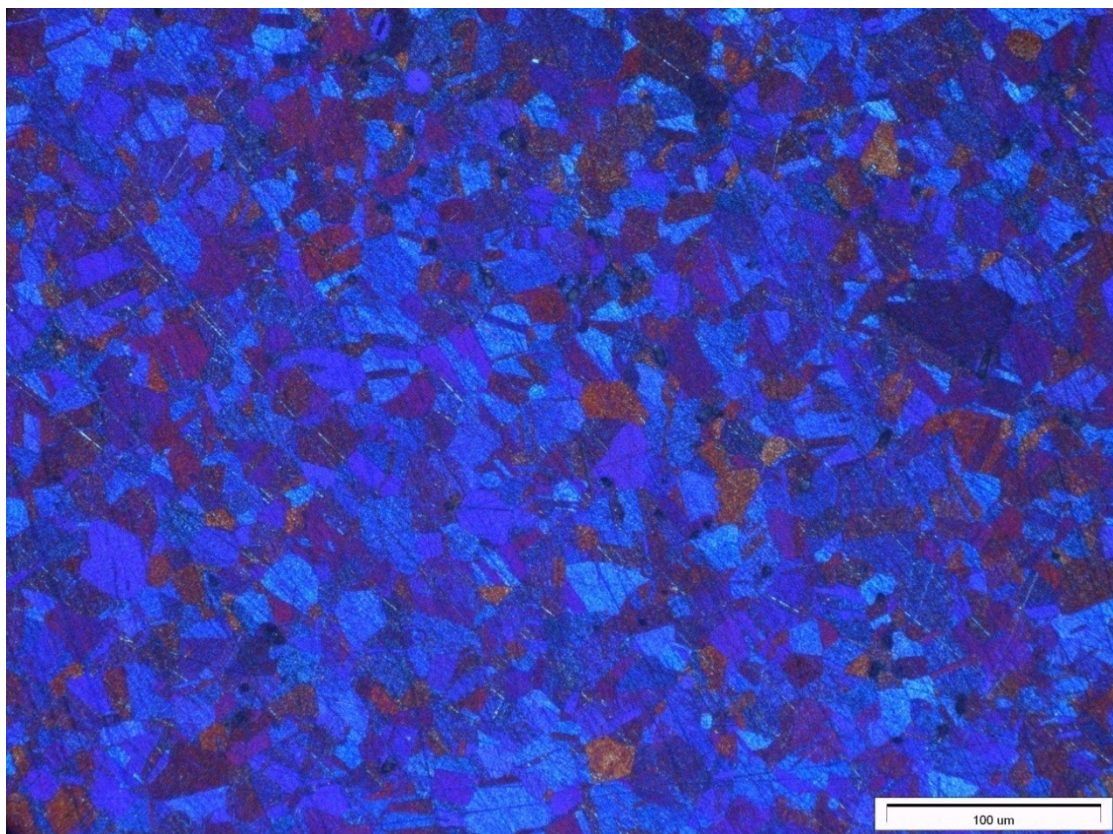
Obrázek: Austenitická ocel BERAHA II polarizované světlo (zvětšeno 250x)
