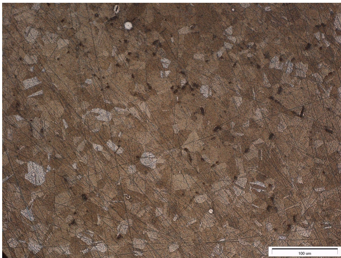
Obrázek: Austenitická ocel BERAHA II (zvětšeno 250x)
