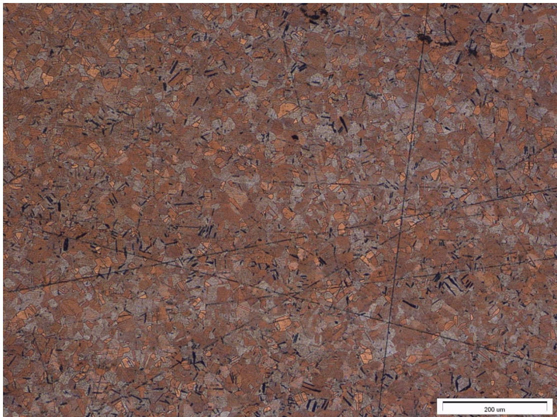
Obrázek: Austenitická ocel BLOECH A WEDL I (zvětšeno 125x)
