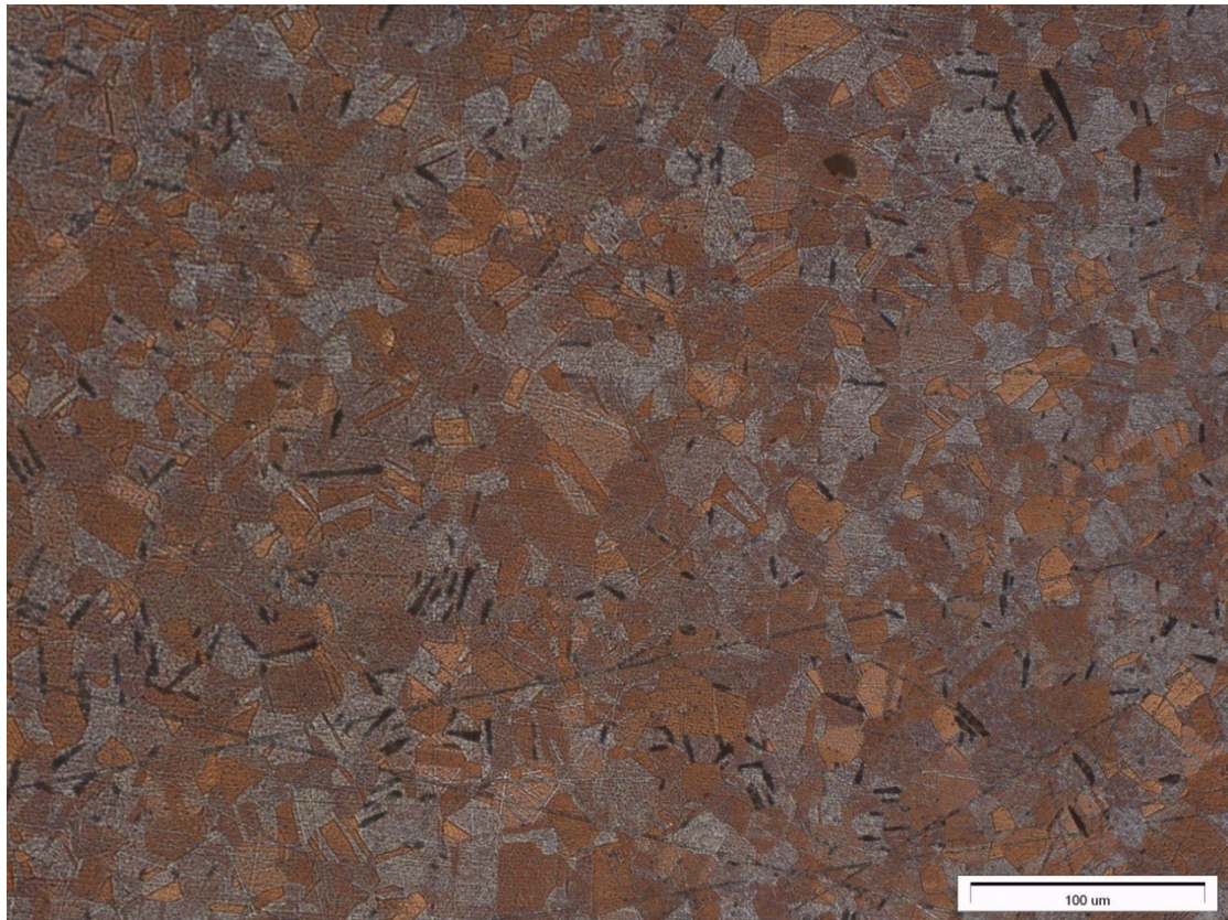
Obrázek: Austenitická ocel BLOECH A WEDL I (zvětšeno 250x)
