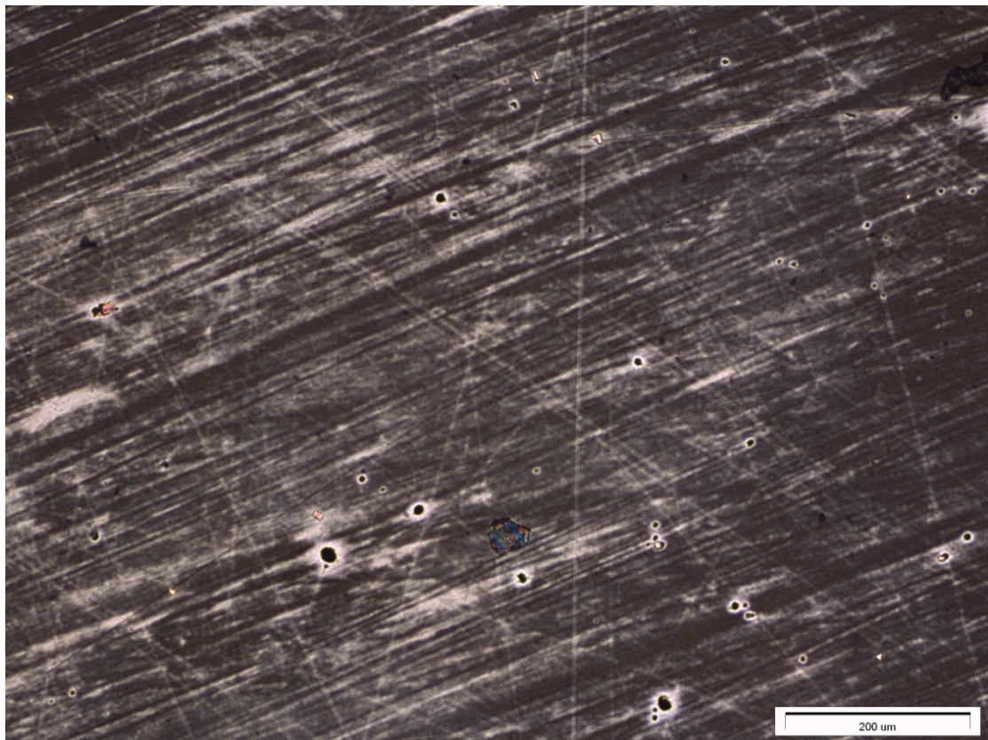
Obrázek: Hadfieldská ocel KLEMM (zvětšeno 125x)
