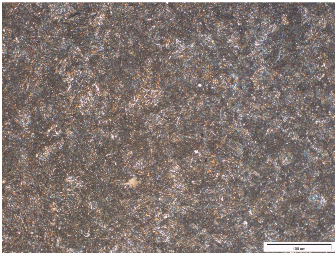
Obrázek: Tepelně zpracovaná ocel 2 BERAHA II (zvětšeno 250x)
