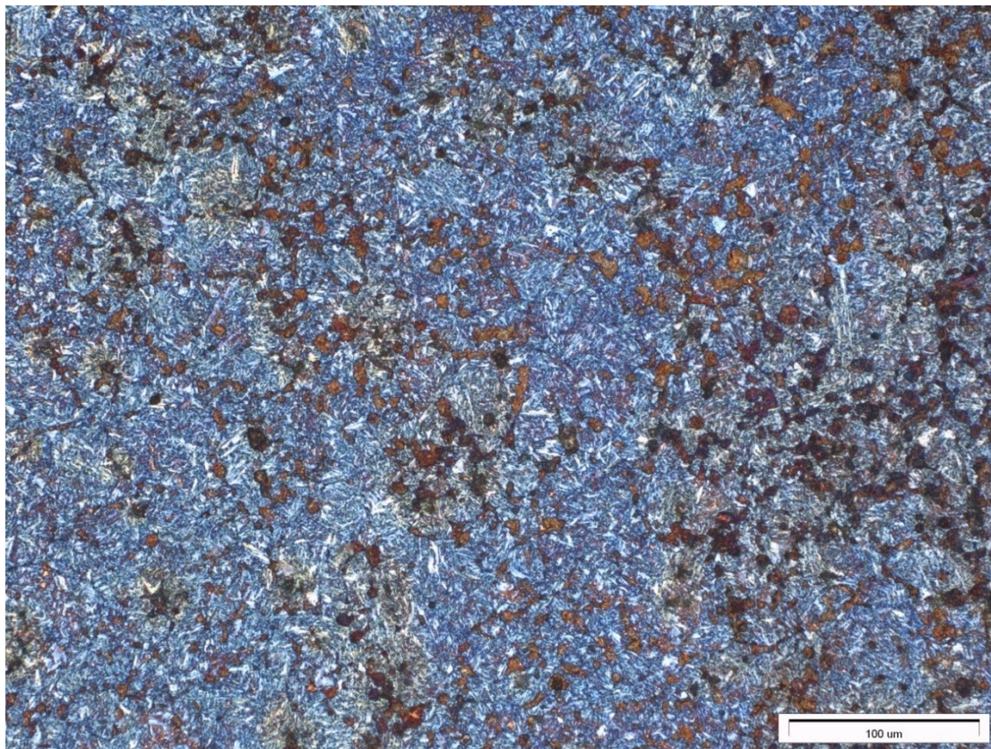
Obrázek: Martenziticko-bainitická struktura BERAHA I (zvětšeno 250x)
