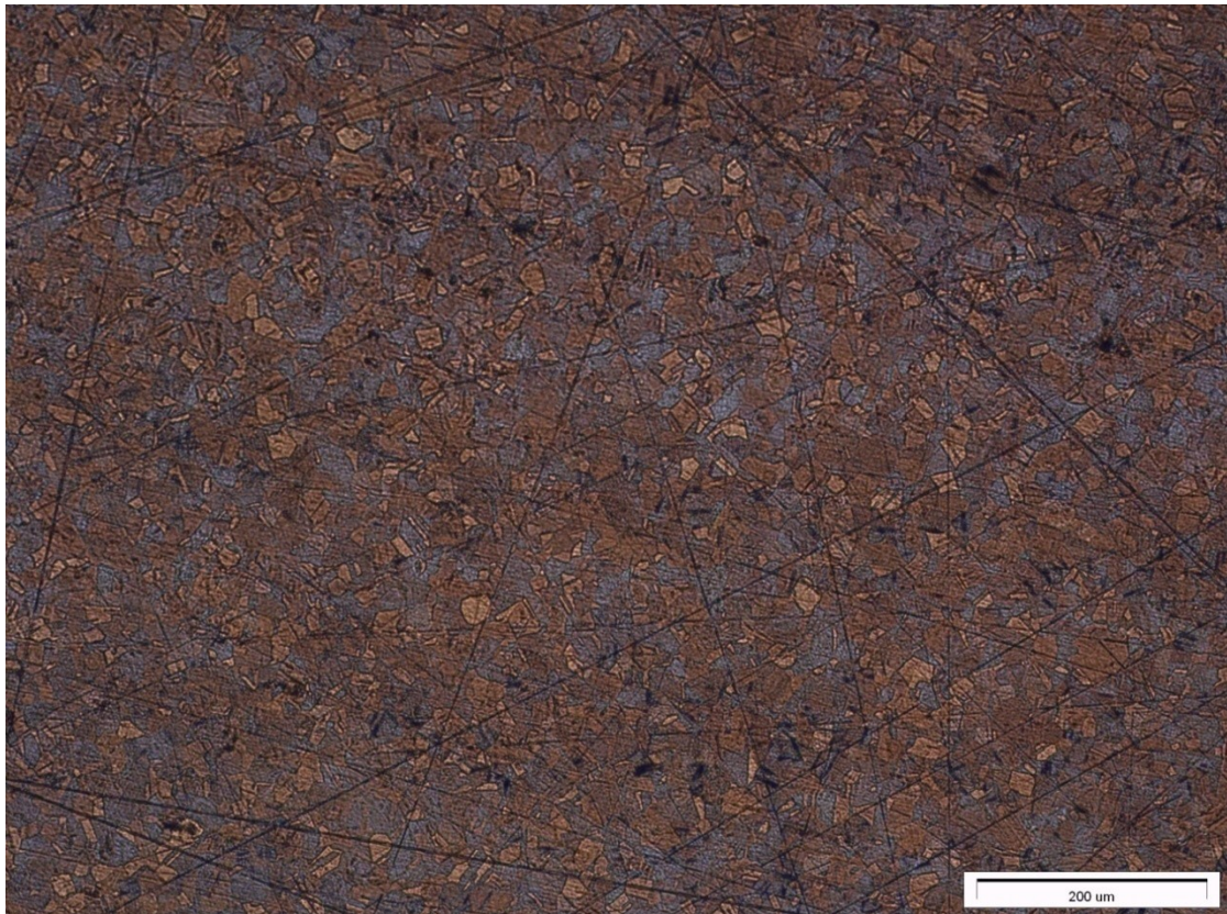
Obrázek: Austenitická ocel 2 BLOECH A WEDL I (zvětšeno 125x)
