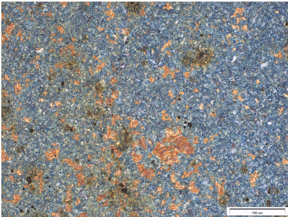
Obrázek: Martenziticko-bainitická struktura 2 BERAHA I (zvětšeno 250x)
