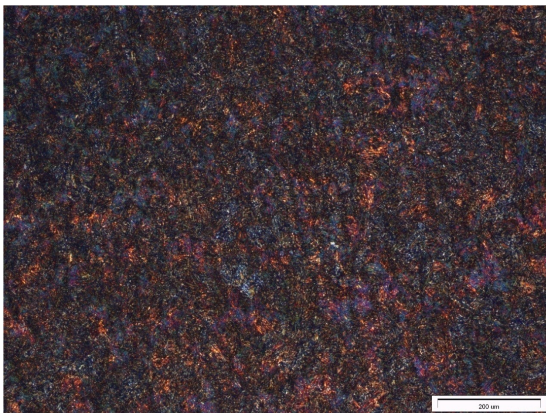
Obrázek: Tepelně zpracovaná ocel BERAHA-MARTENZIT (zvětšeno 125x)
