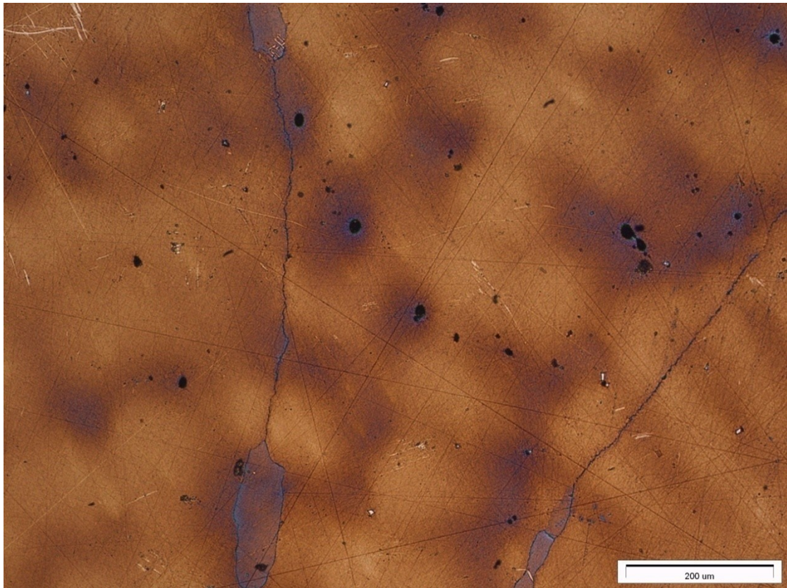
Obrázek: Hadfieldská ocel NITAL (zvětšeno 125x)
