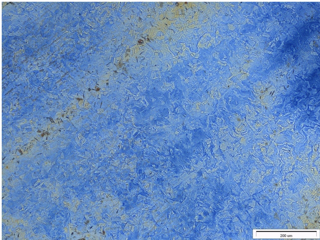
Obrázek: Austenitická ocel LICHTENEGGER A BLOECH I (zvětšeno 125x)
