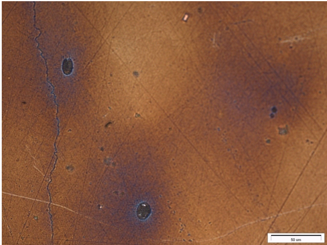
Obrázek: Hadfieldská ocel NITAL (zvětšeno 400x)
