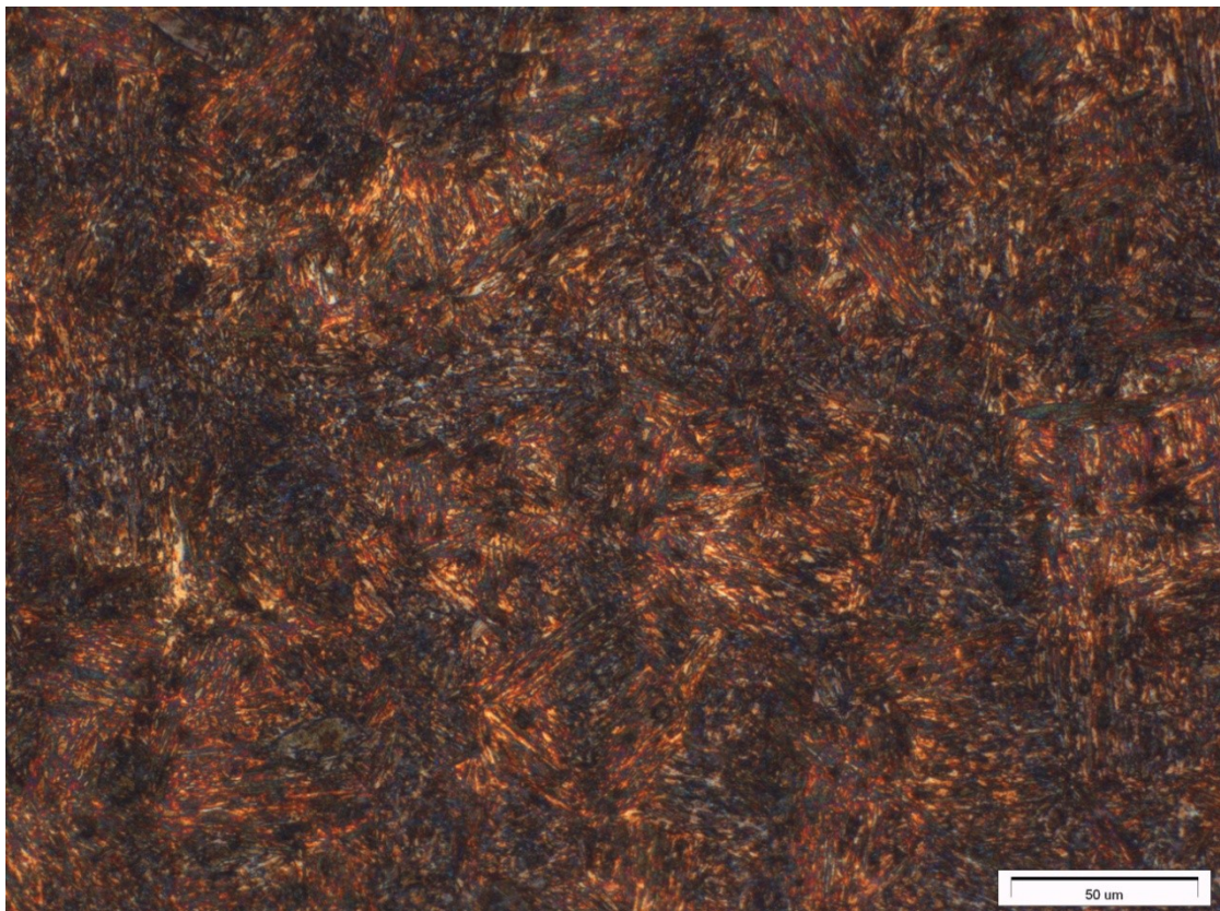
Obrázek: Tepelně zpracovaná ocel BERAHA-MARTENZIT (zvětšeno 400x)
