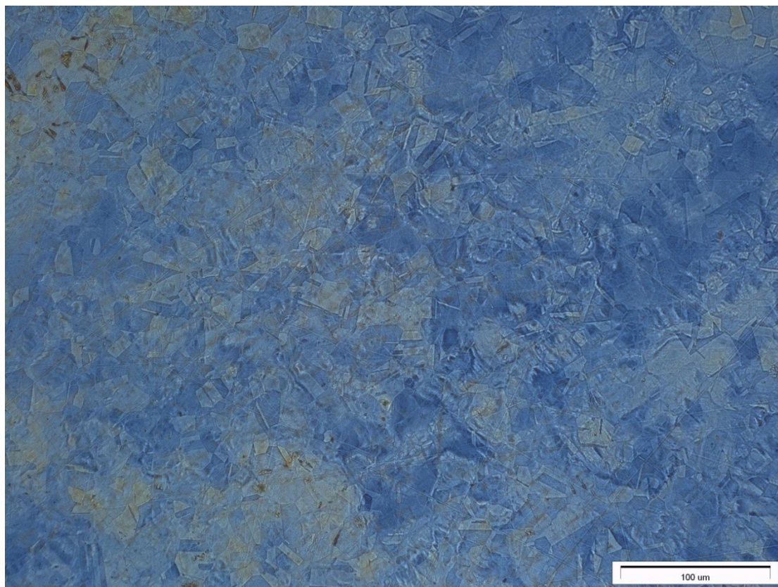
Obrázek: Austenitická ocel LICHTENEGGER A BLOECH I (zvětšeno 250x)
