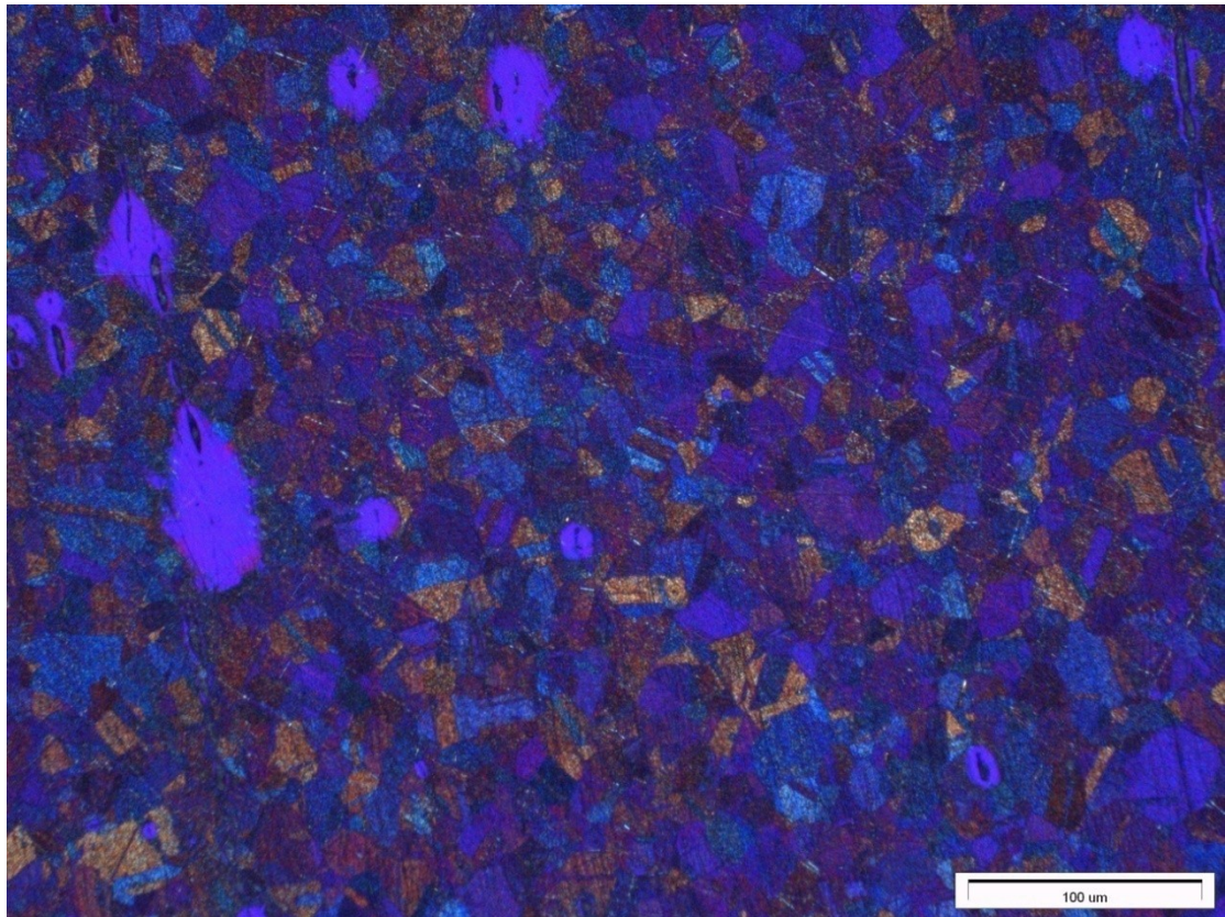
Obrázek: Austenitická ocel 2 BERAHA II polarizované světlo (zvětšeno 250x)
