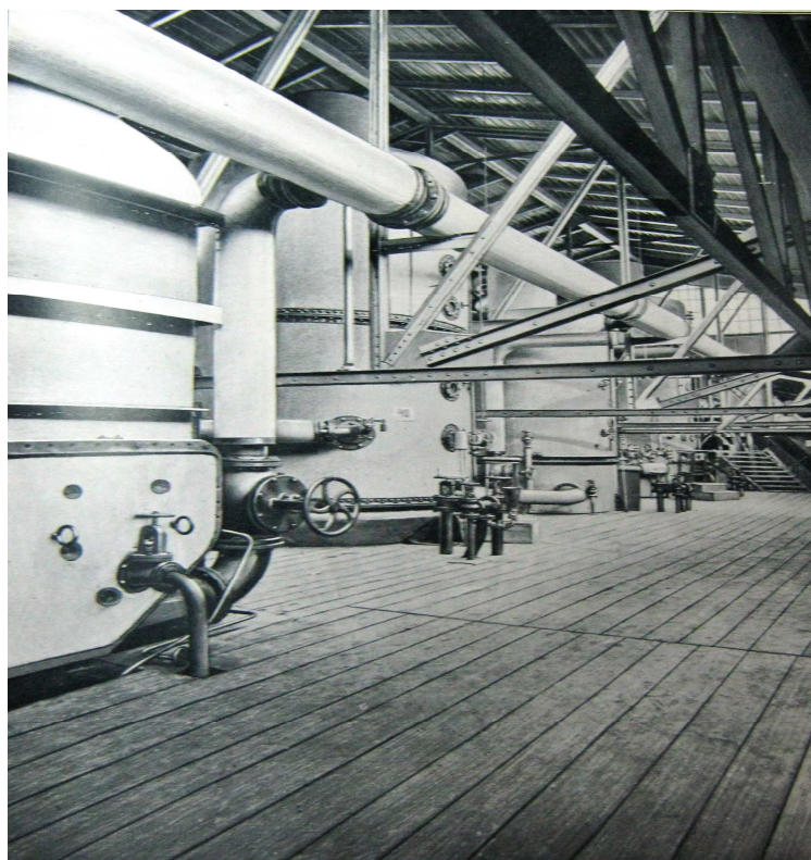
Obrázek č. 10 – vakuová stanice
