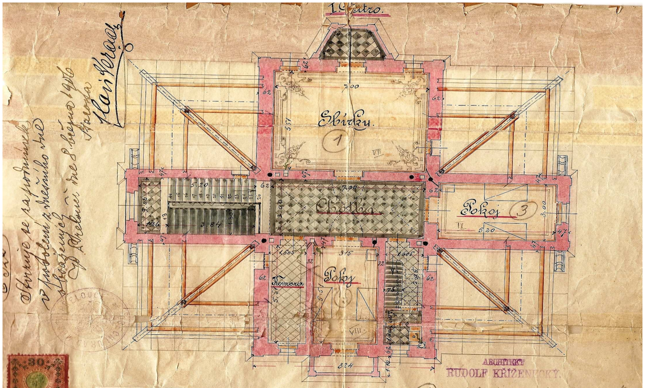
Obrázek č. 22 – stavební plány Divišovy vily (1. patro)
