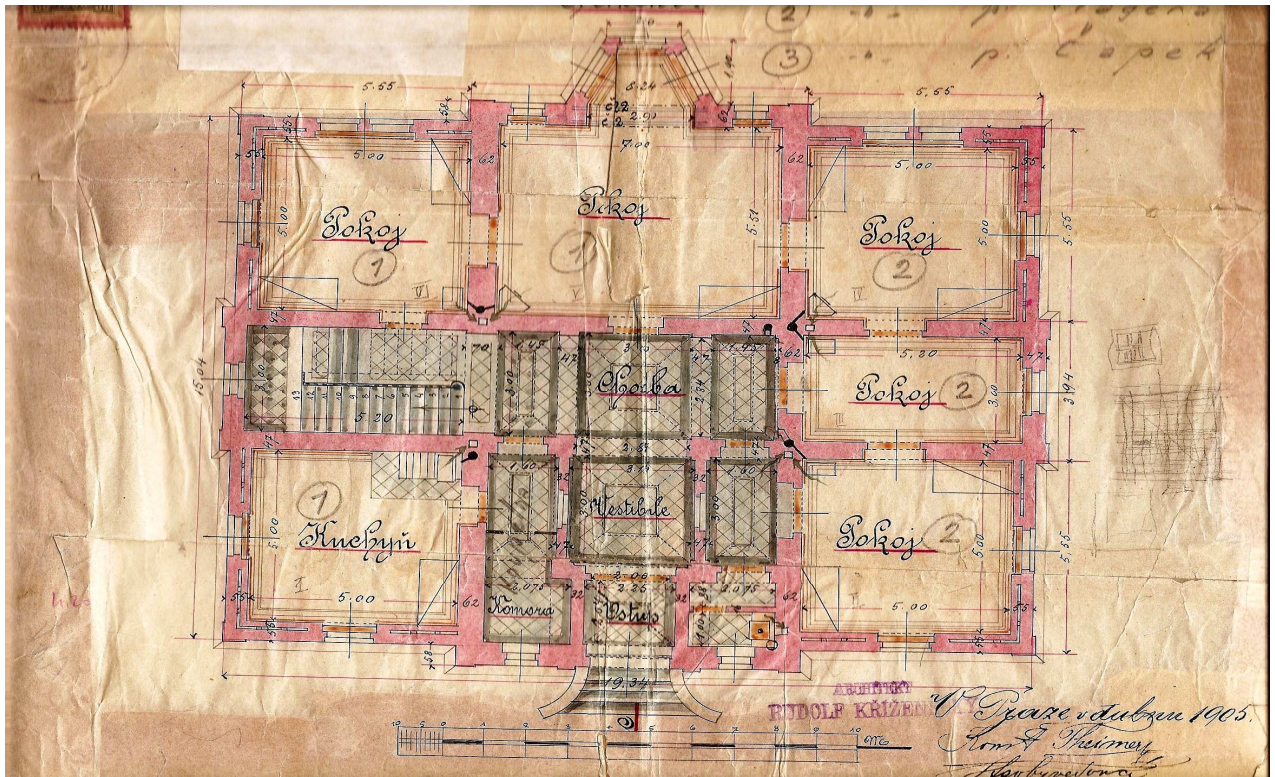
Obrázek č. 22 – stavební plány Divišovy vily (1. patro)
