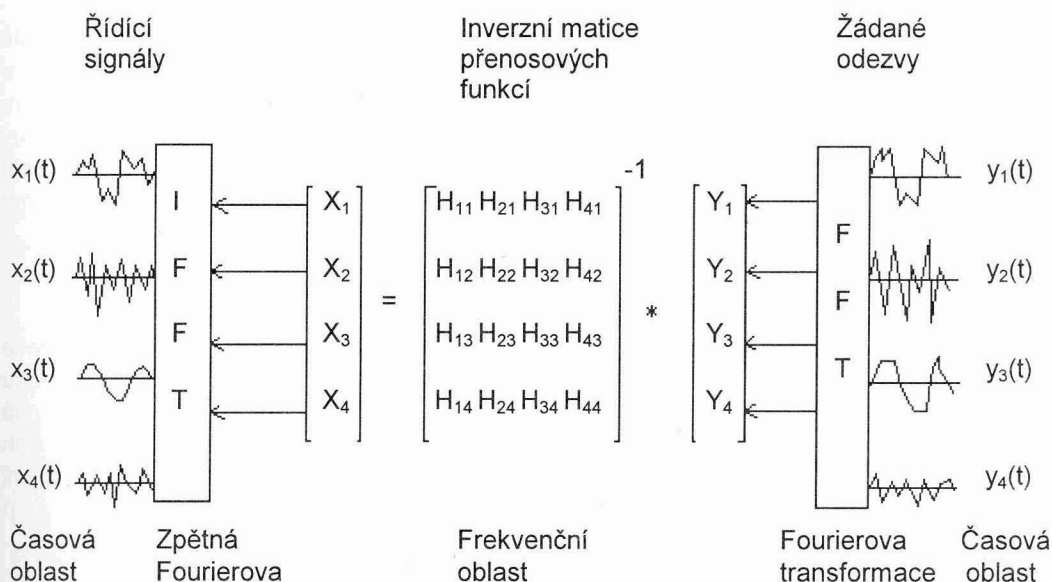
Obr. 2 Schematické znázornění procesu iterace řídicích signálů
