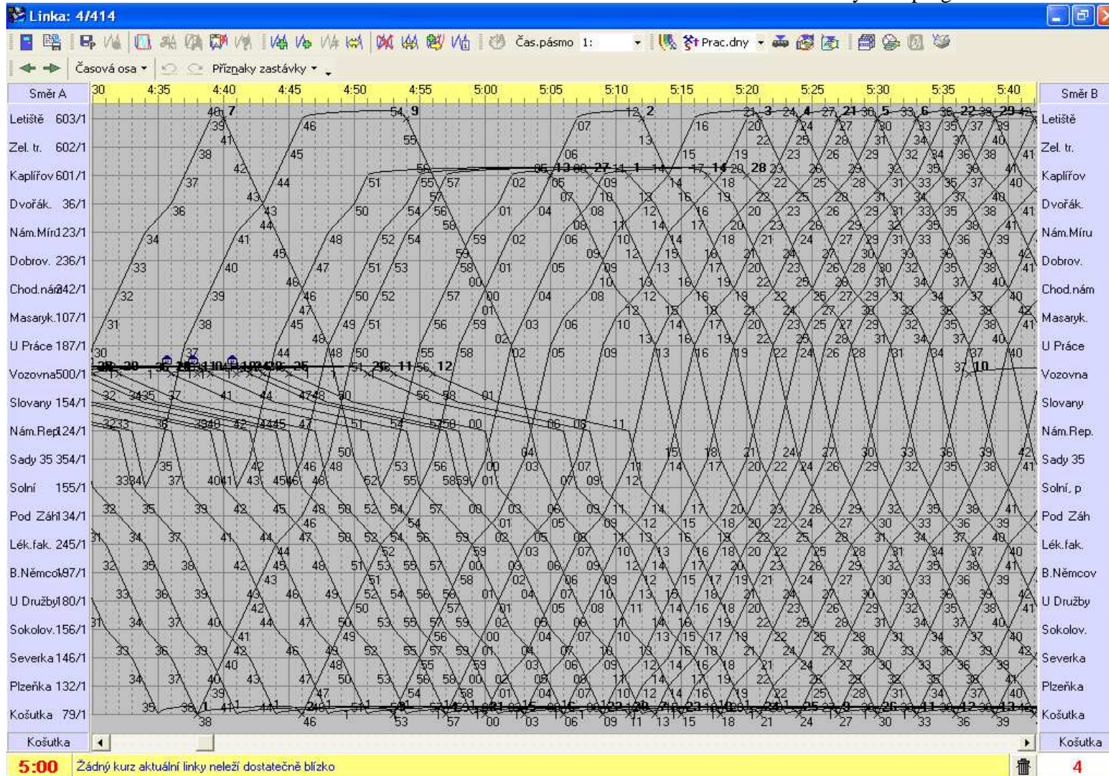
Příloha č. 18 – výřez z programu FS Grafikon, linka č. 4.
