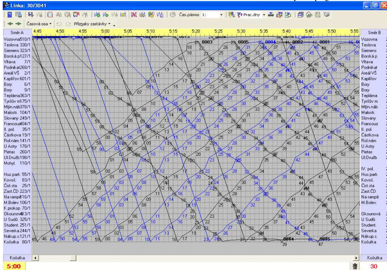
Příloha č. 19 – výřez z programu FS Grafikon, linka č. 30.
