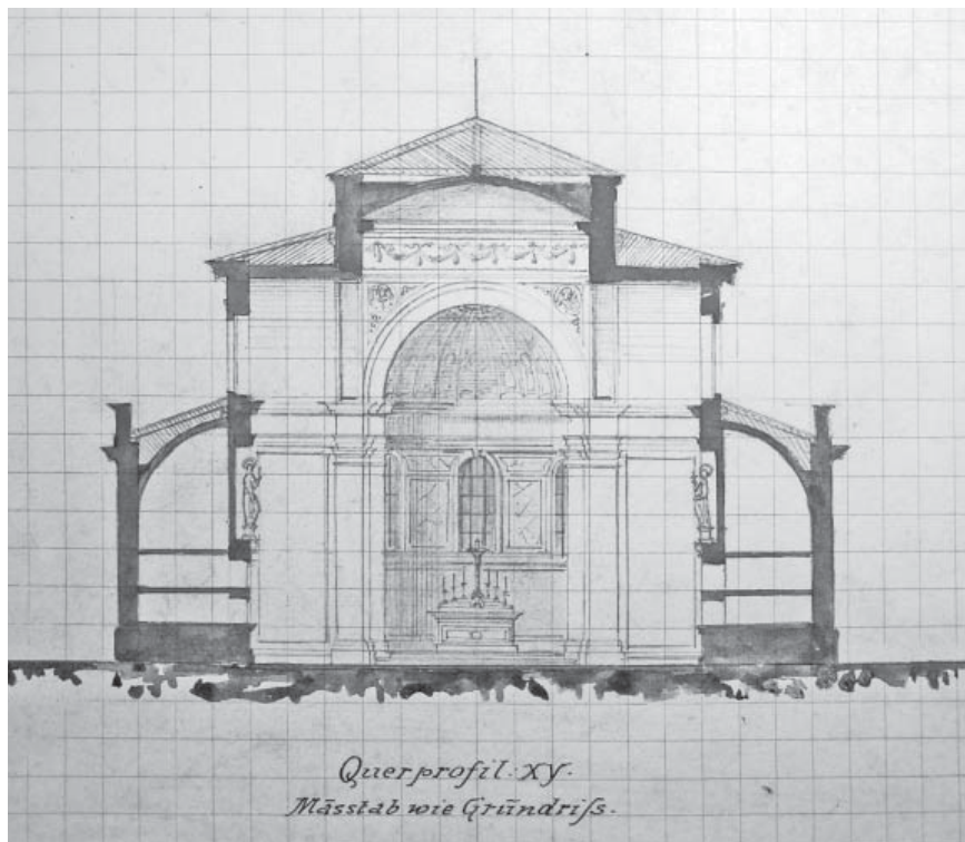
Nerealizovaný návrh na přestavbu kaple sv. Marka v Cholenicích, počátek 20. století.
